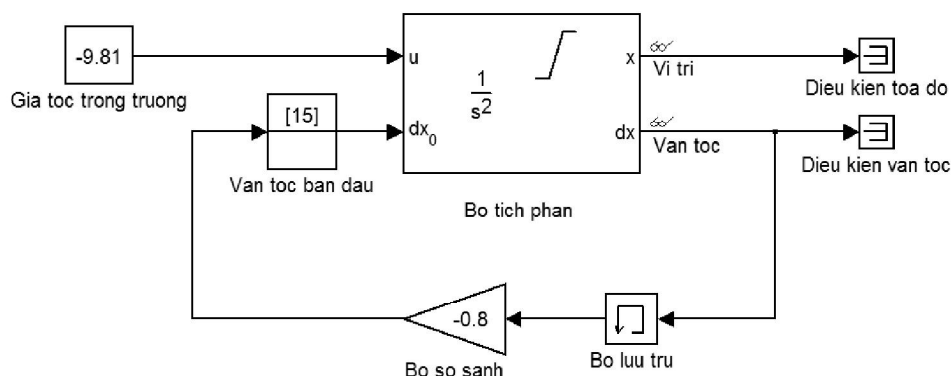
Hình 2. Sơ đồ khối giải bài toán chuyển động của quả bóng cao su bằng Simulink
