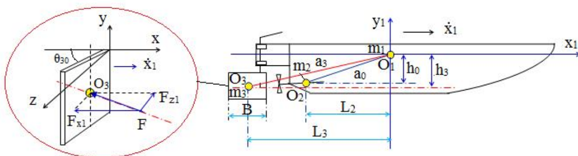
Hình 2. Sơ đồ xác định lực tác dụng lên xuồng chứa cháy khi quay vòng
