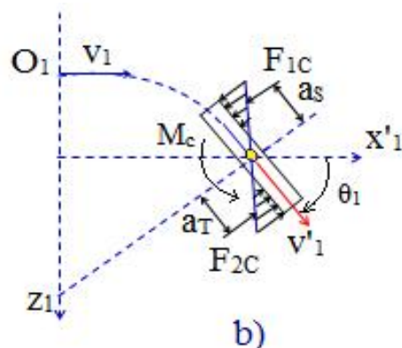
Hình 3. Sơ đồ xác định các thông số động học và lực cản khi xuồng quay vòng
