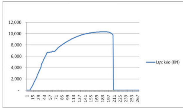
Hình 08. Số liệu đo sau khi lưu thành file dữ liệu và vẽ lại trên excel
