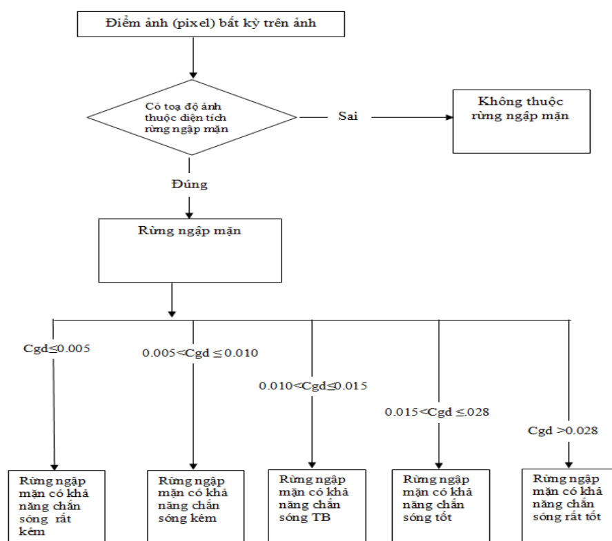
Hình 7. Sơ đồ bộ khoá giải đoán khả năng chắn sóng của rừng ngập mặn
