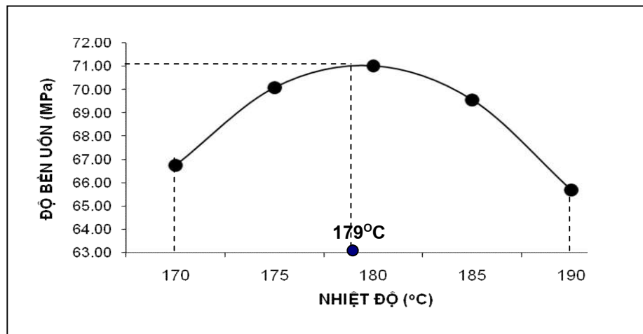
Hình 06. Đồ thị ảnh hưởng của nhiệt độ ép đầu vôi phun tới độ bền uốn
